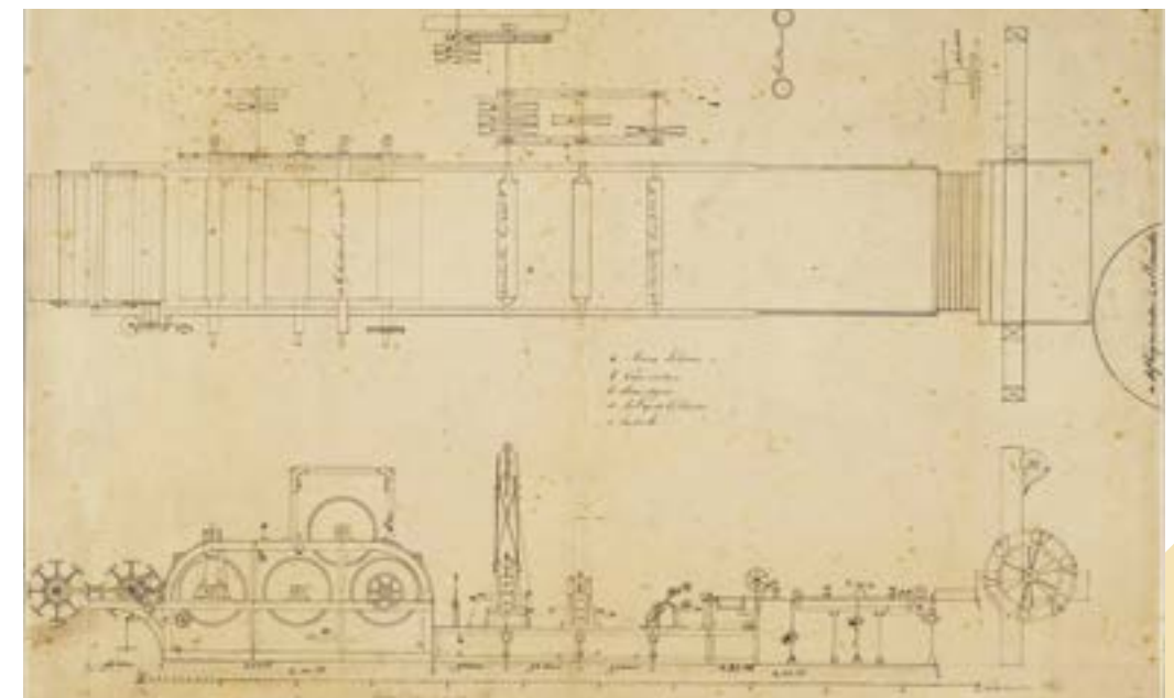
Tekening van een papiermachine, jaartal onbekend, in 1928 geschonken aan De Zaanse Molen; mogelijk stond deze machine in Het Fortuin
